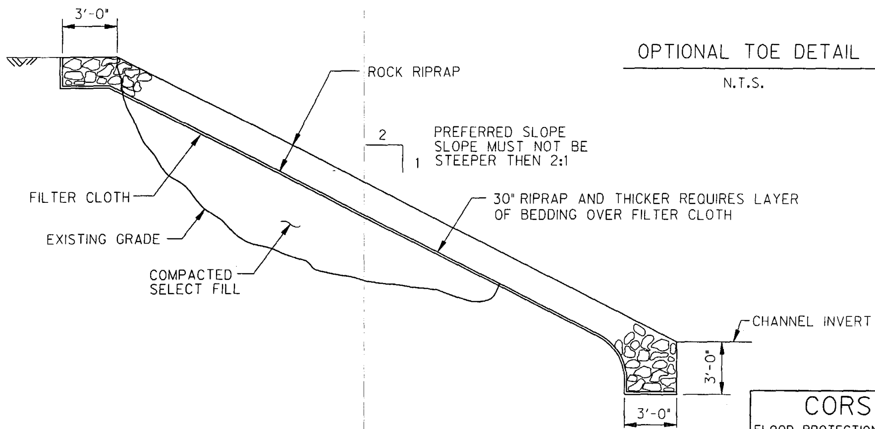
TYPICAL ROCK RIPRAP SECTION N.T.S.
