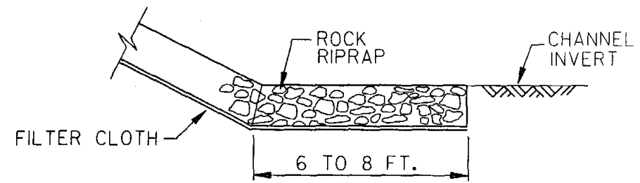
OPTIONAL TOE DETAIL N.T.S.
