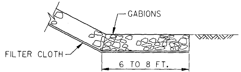
OPTIONAL TOE DETAIL
